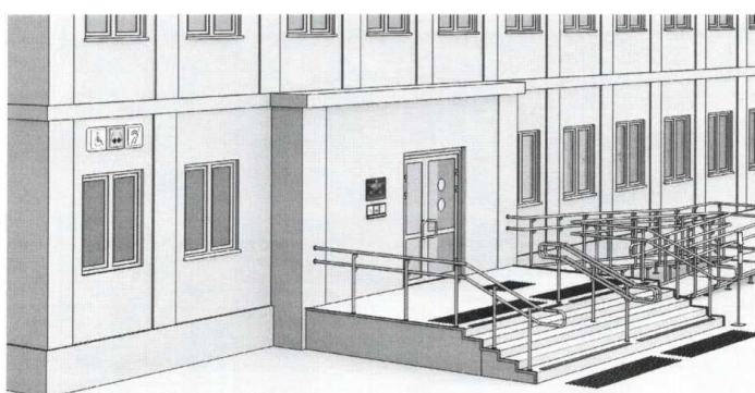
Рисунок А.2 — Пример размещения светозвукового маяка на фасаде здания на высоте 4,5 м для обозначения доступности объекта
