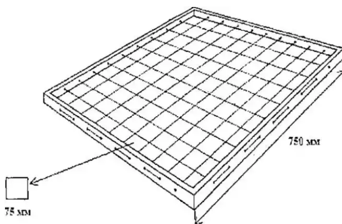
Рисунок 3 - Рама для измерения плотности травяного покрова
