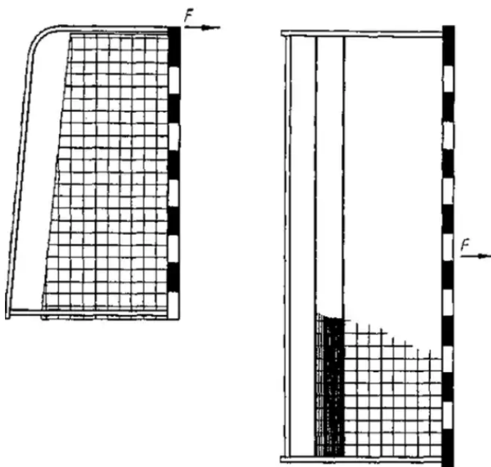
Рисунок 12 - Проверка стабильности ворот для мини-футбола
