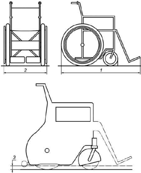
1 - максимальная длина; 2 - максимальная ширина; 3 - минимальный дорожный просвет
