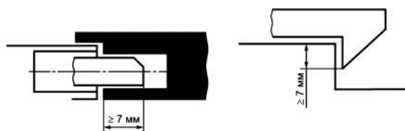
Рисунок 10 - Пример запирающего элемента
