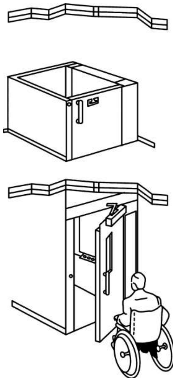
Рисунок 7 - Пример вертикальной платформы с огражденной шахтой
