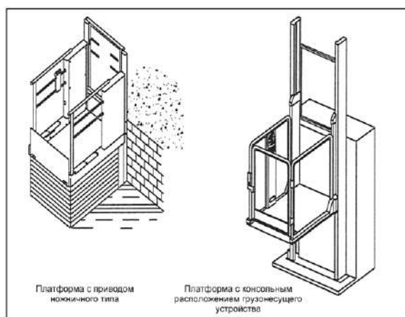
Рисунок 1 — Примеры вертикальных подъемных платформ с неогражденной шахтой
