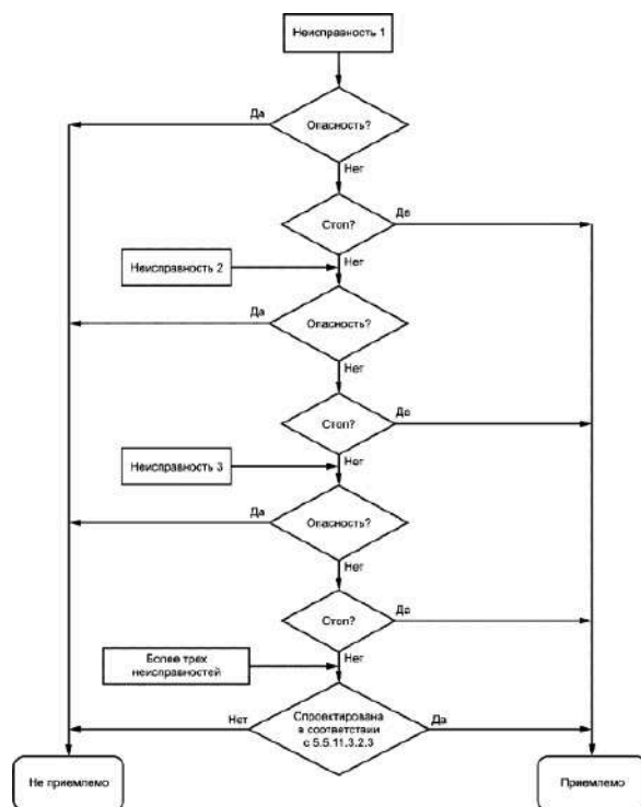
Рисунок 5 - Блок-схема оценки цепи безопасности
