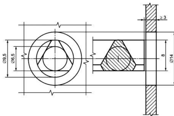
Рисунок 11 - Треугольная ключевина
