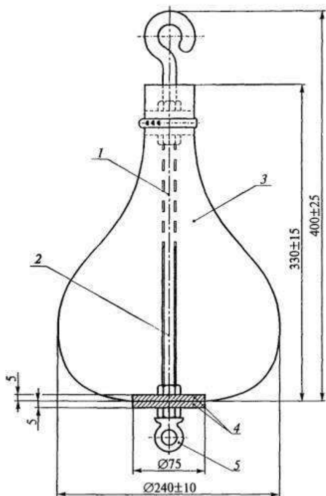
Рис. 3 . Маятник для нежесткого удара:
