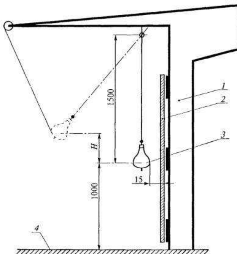
Рис. 1 . Испытательный стенд:
