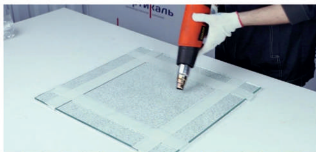
ЭТАП #1 Прогреваем поверхность пола и плитки
