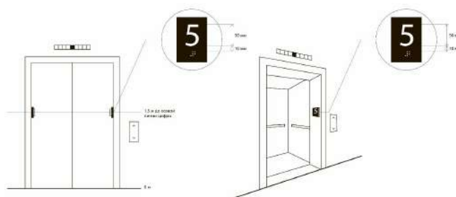
Рисунок 10 — Обозначения номера этажа на боковых поверхностях дверных проемов лифтовой шахты
