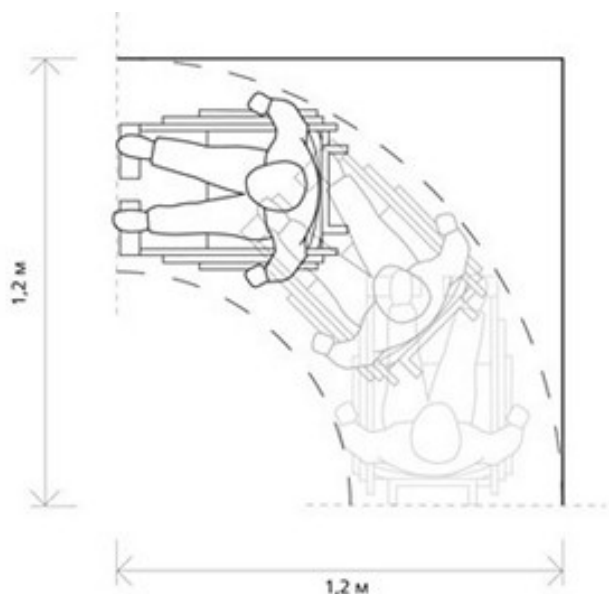
Рисунок Б.2 — Пространство для поворота на 90^\circ
