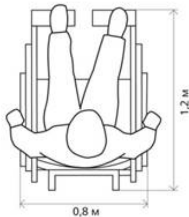
Рисунок Б.1 — Габариты кресла-коляски
