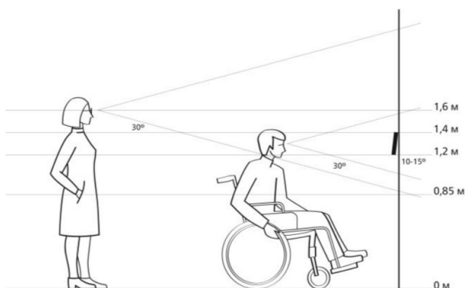
Рисунок 15 — Высота размещения информации для инвалида, использующего для передвижения
