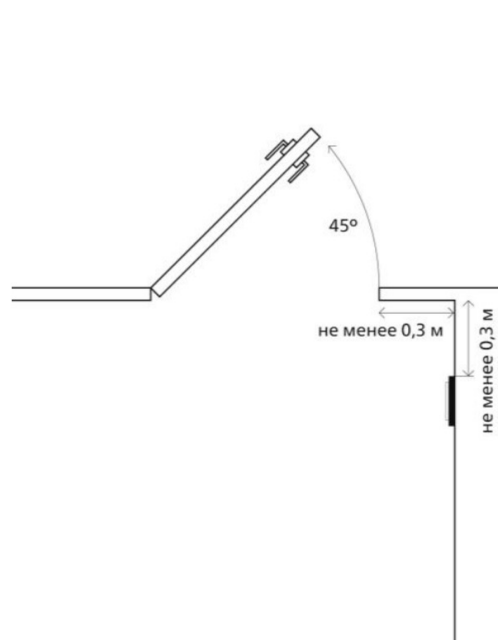
Рисунок 10 — Размещение информации при угловом расположении двери при затесненных условиях
