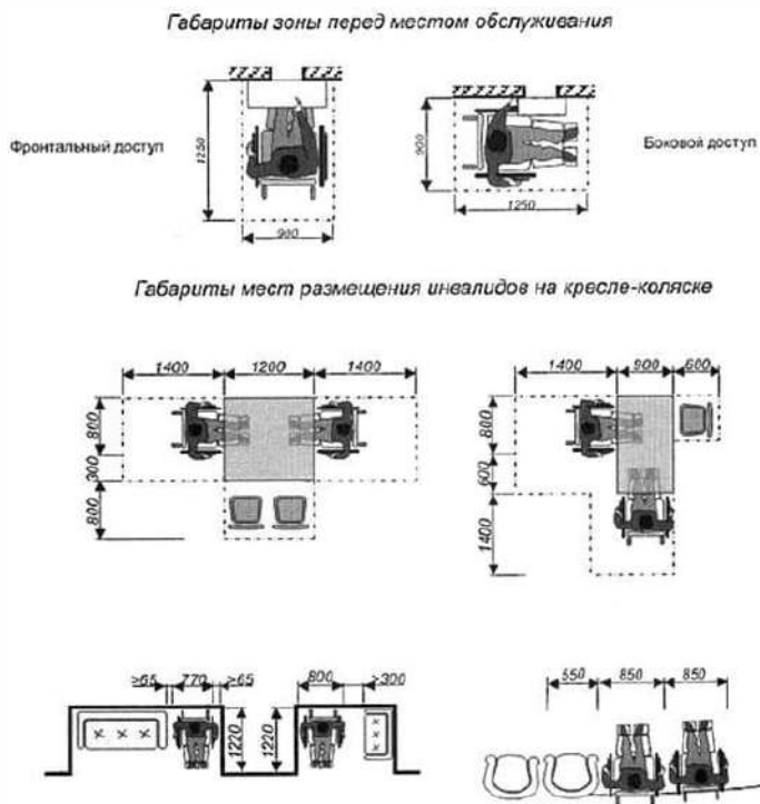
Минимальные размеры свободного пространства для доступа к сиденьям и столам
