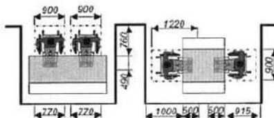
Рисунок Г.5 - Габариты у мест обслуживания
