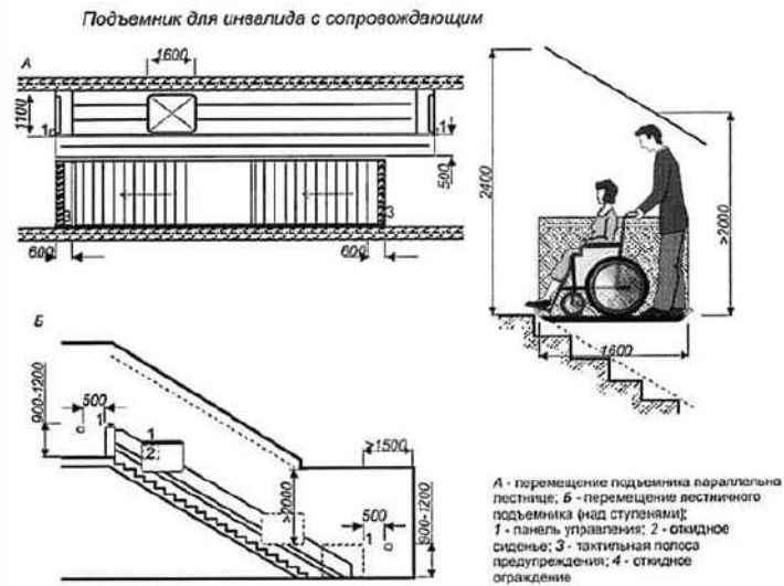
Подъемник для самостоятельного перемещения инвалида
