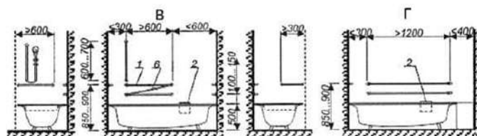
Поручни в кабинках с ванными для "сидячих" (В) и "лежачих" (Г) инвалидов
